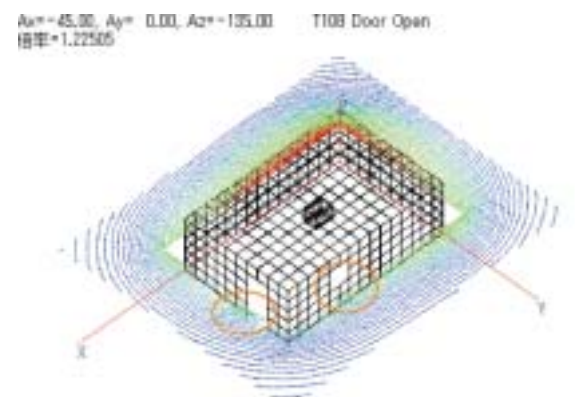
図5 シールドルームのドアと窓から漏れ出す磁場・鳥瞰図
