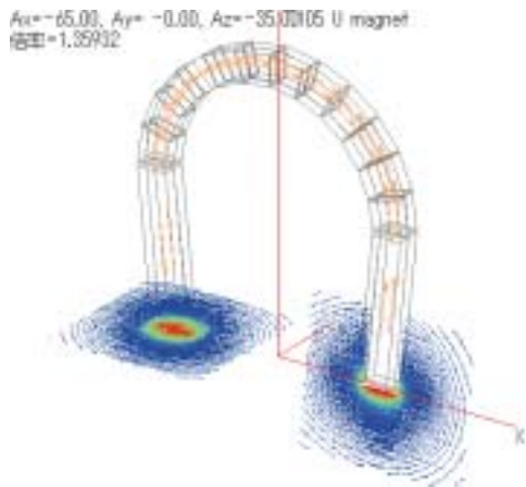
図2 馬蹄形磁石が作る磁場
