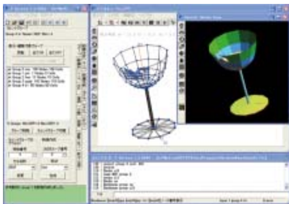
図6 3次元プリプロセッサP
