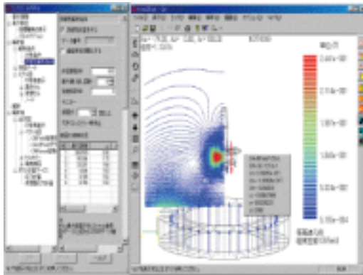
図1 3次元リアルタイム磁場解析ソルバ-Qm (図は宙に浮く独奏の解析)
