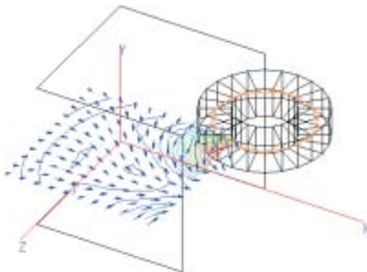
図3 ベースポール型コイルとギャップのあるリングヨークが作る磁場
