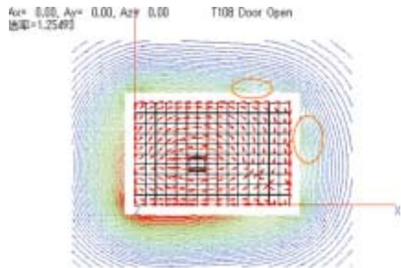
図4 シールドルームのドアと窓から漏れ出す磁場・平面図
